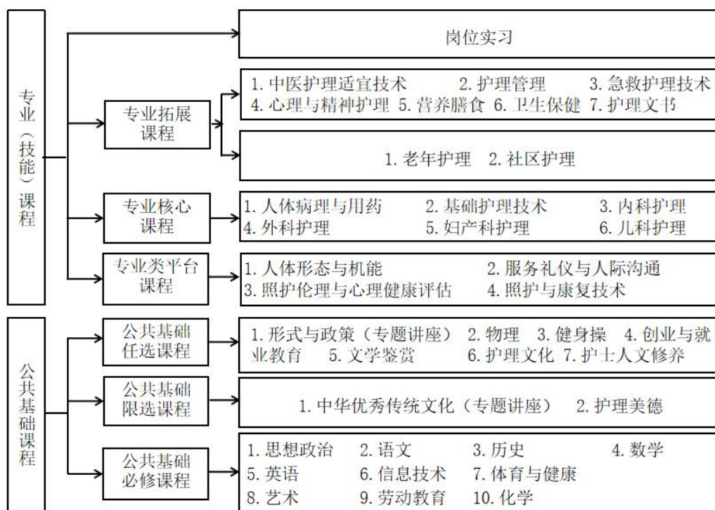
图1 课程结构图
